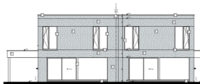
Achteraanzicht
