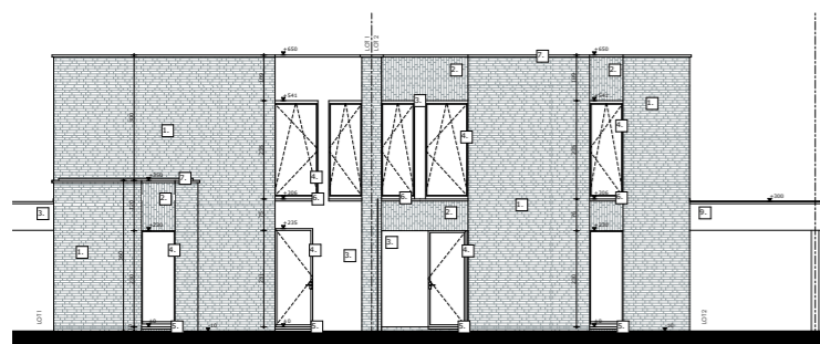
Vooraanzicht
