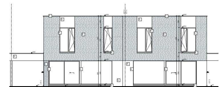
Achteraanzicht
