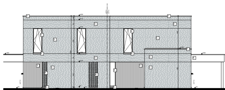
Vooranzicht
