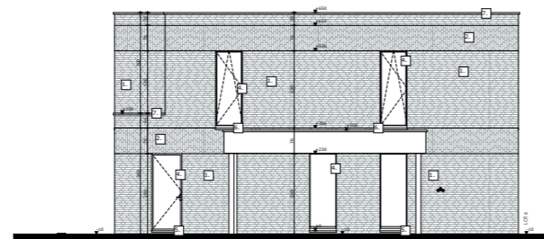
Rechteraanzicht
